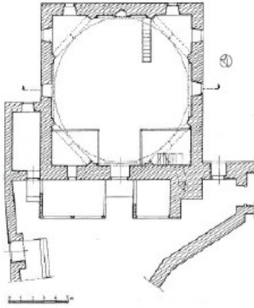
Çizim 1: Selim Ağa Camisi planı (K.Pektaş'tan) (K.Pektaş'tan)
