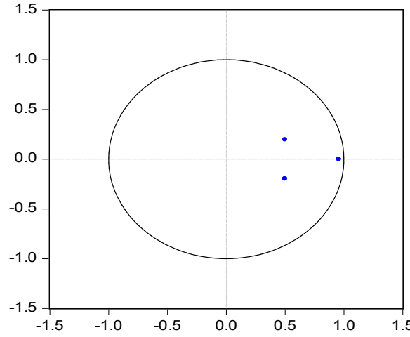
Grafik 1: AR Karakteristik Polinomun Ters Köklerine Ait Birim Çember Inverse Roots of AR Characteristic Polynomial
