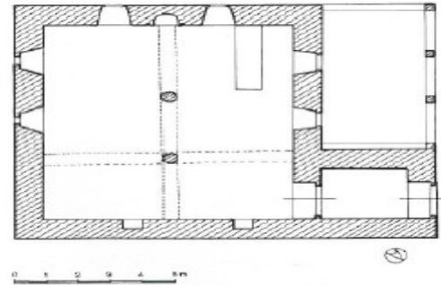
Çizim 4: Dolunay Köyü camisi planı (K.Pektaş'tan)
