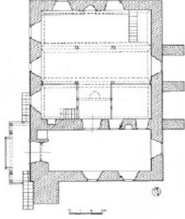
Çizim 5: Yeşilyurt Köyü Camisi planı (K.Pektaş'tan)
