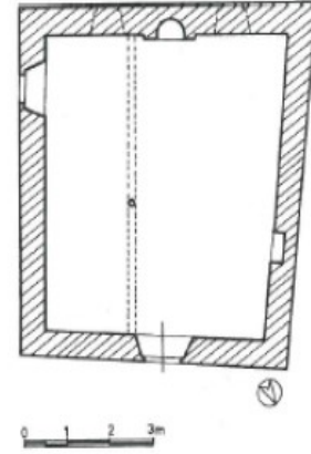
Çizim 2: Müftüoğlu Camisi planı
