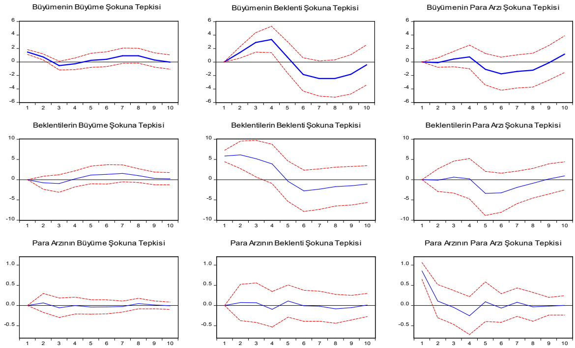
Grafik 1: Etki-Tepki Fonksiyonlarının Grafiksel Gösterimi
